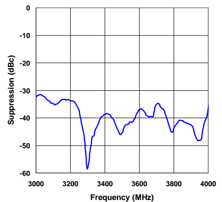
Sideband Suppression
